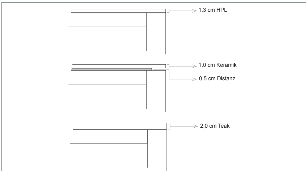
Aufbau der Tischplatten in HPL | Keramik | Teak
