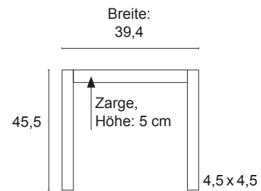
Seitenansicht (Stirnseite)
