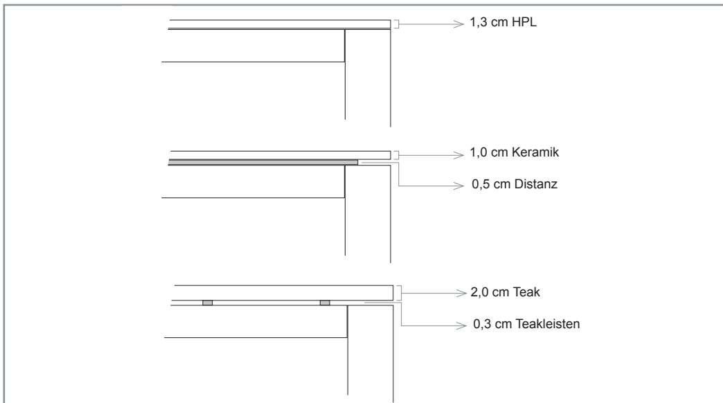
Aufbau der Tischplatten in HPL, Keramik und Teak
