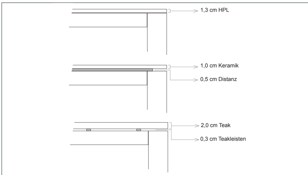
Aufbau der Tischplatten in HPL, Keramik und Teak
