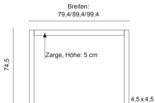
Seitenansicht (Stirnseite)
