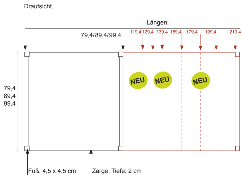
Tisch-Untergestelle
