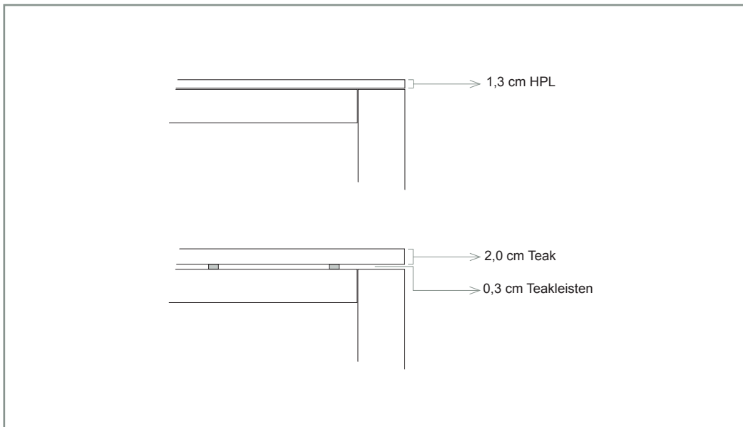
Aufbau der Tischplatten in HPL und Teak
