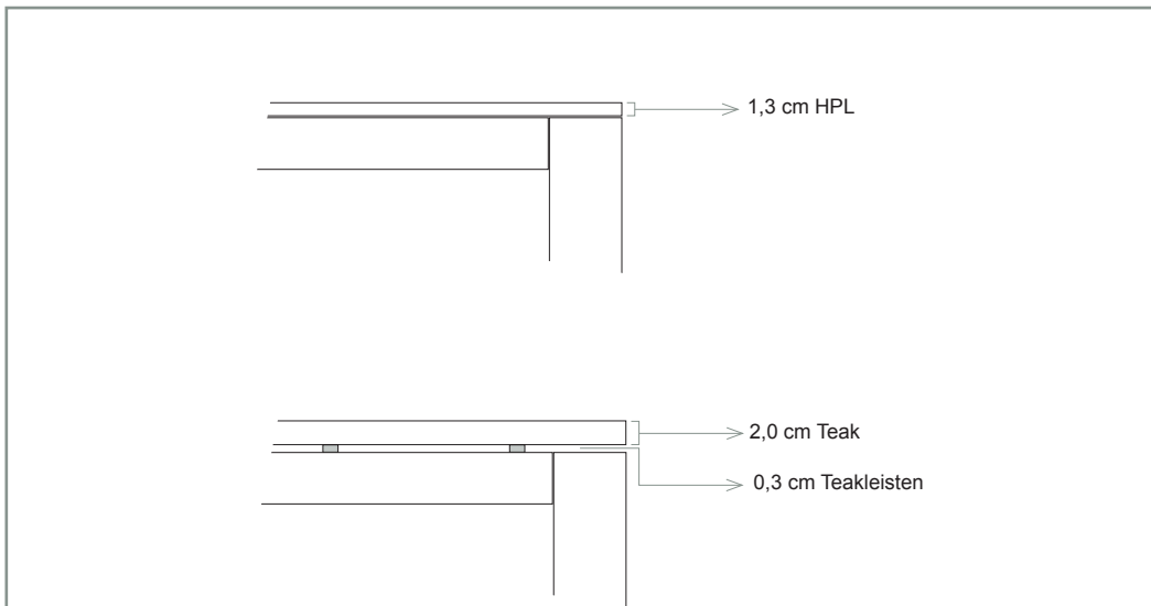
Aufbau der Tischplatten in HPL und Teak
